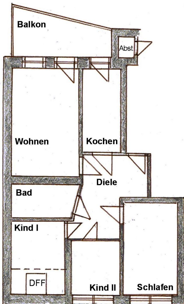
Grundriss
